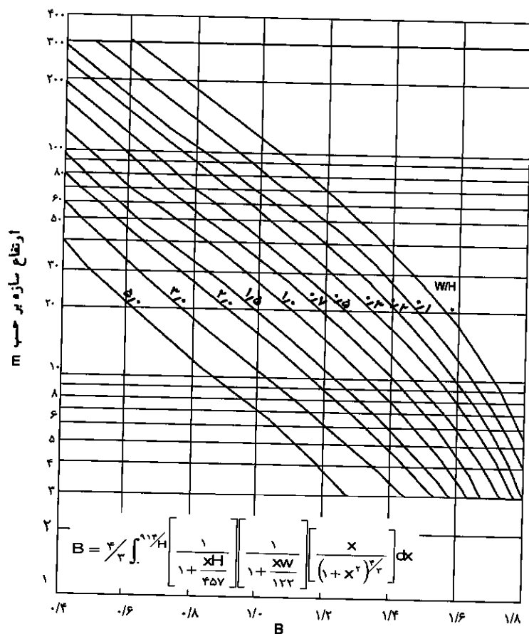
شکل پ-۶-۱ ضریب آشفته‌گی محیط ساختمان (B)
