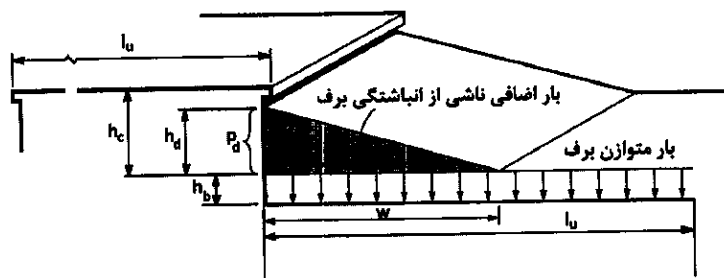
شکل ۷-۶-۸ نمایش برف انباشته شده بر بام پایین‌تر
