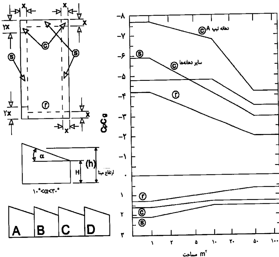
شکل ۱۰-۱۰-۶- ضرایب ترکیبی فشار و مکش خارجی C_p C_g برای طراحی پوشش‌ها و اجزاء بام‌های دندانه‌ای یک‌طرفه
