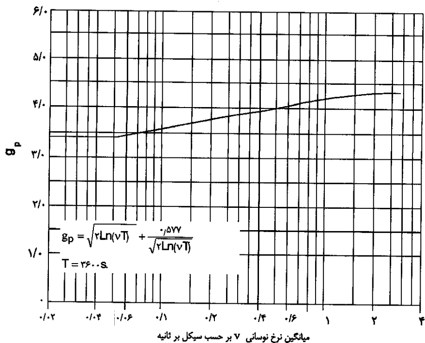
شکل پ-۶-۴ ضریب پیشینه آماری بار ( G_p )
